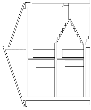
Sezione
